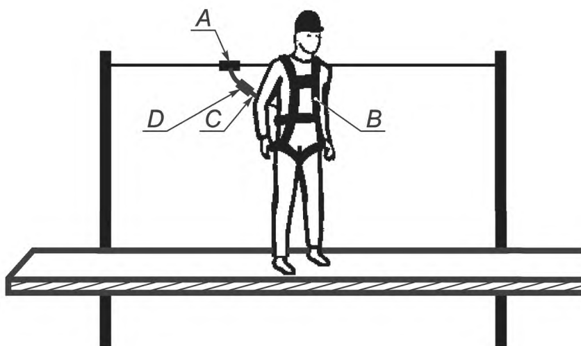
Рисунок 5 — Пример страховочной системы со стропом и амортизатором
