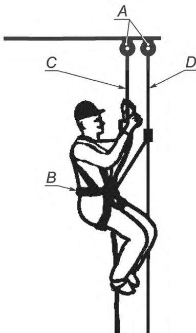
A — анкерная точка; B — привязь; C — рабочий канат; D — страховочный канат
