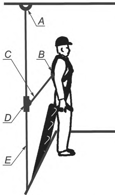
A — анкерная точка; B — страховочная привязь; C — строп; D — устройство ползункового типа; E — гибкая анкерная линия
