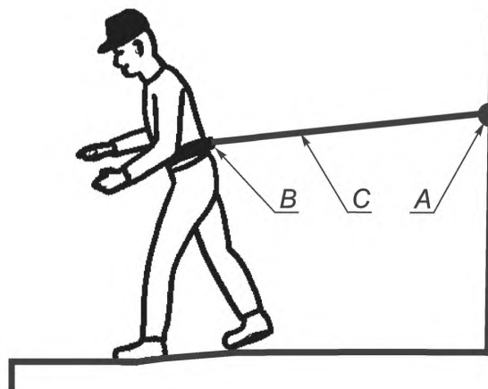
А — анкерная точка; В — привязь; С — строп
