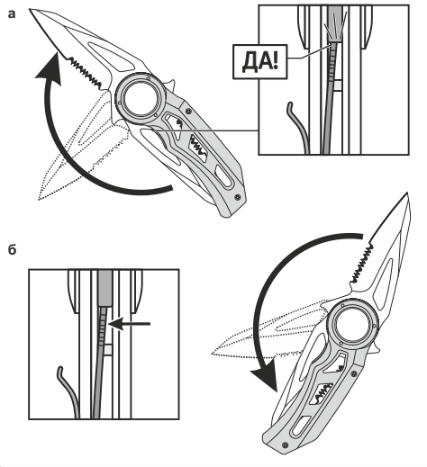
Рис. 2. Принцип работы
