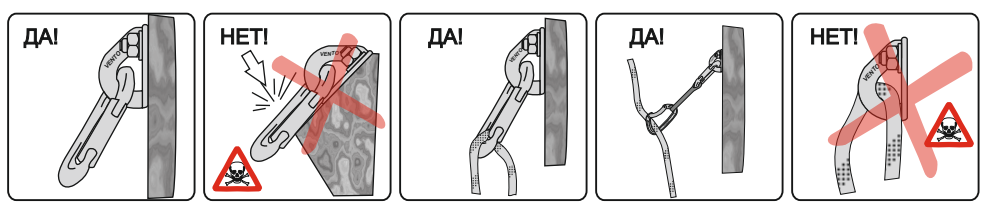
Рис. 6. Положение анкерного устройства и карабина
